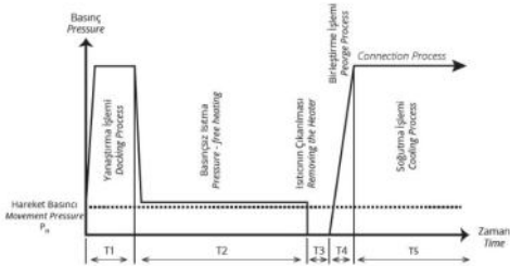
ALIN KAYNAK İŞLEMİNİN GRAFİKLE GÖSTERİMİ THE GRAPHIC OF BUTT WELDING PROCESS
