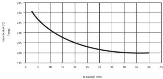
ET KALINLIĞINA GÖRE SICAKLIK DEĞERLERİ TEMPERATURE VALUES ACCORDING TO WALL THICKNESS
